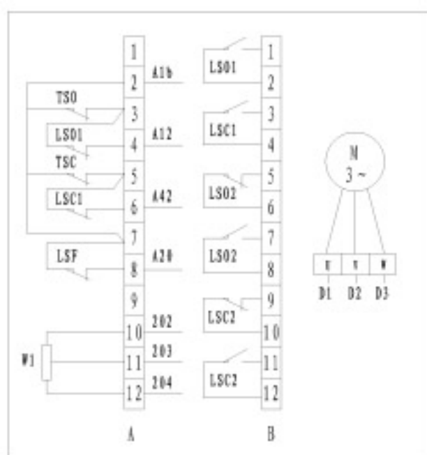
Z 系列常规户外型端子接线图
