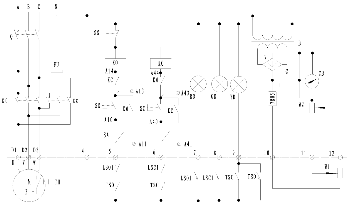
Q 系列常规型电气原理图
