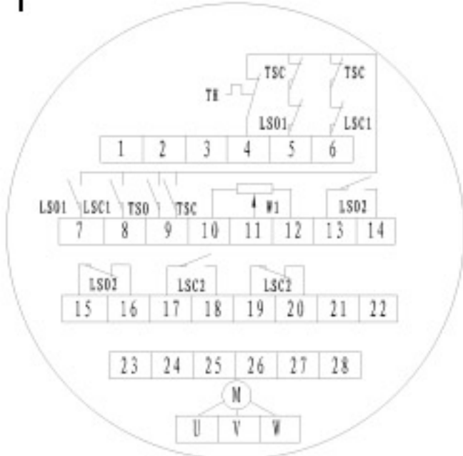
Q 系列常规户外型端子接线图
