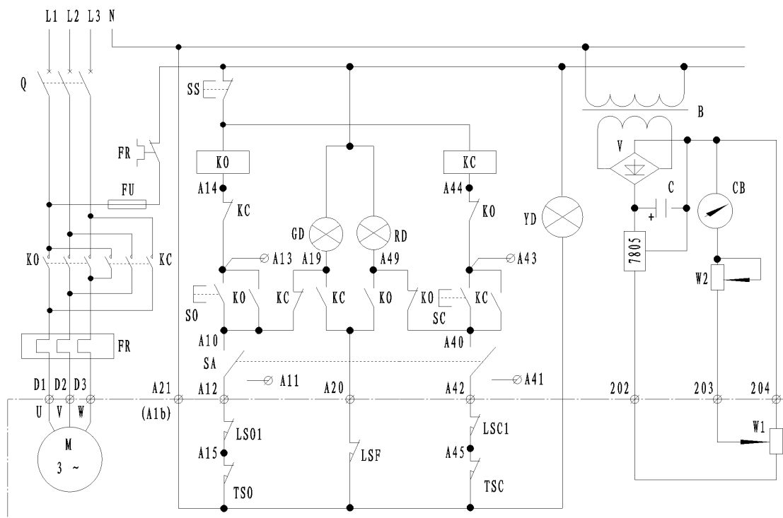
Z 型控制箱电气原理图
